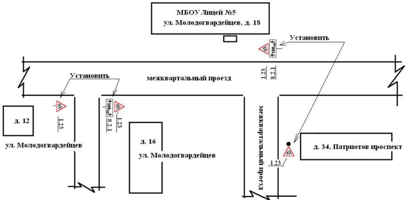
Схема организации дорожного движения в районе месторасположения МБОУ Лицей №5 ул. Молодогвардейцев, д. 18 управа Советского района
